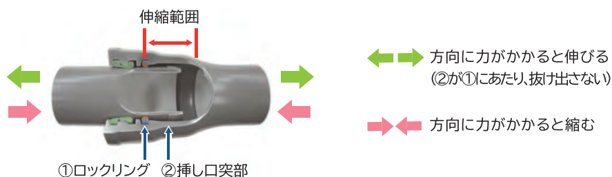
抜け出し防止機能を有する耐震継手
